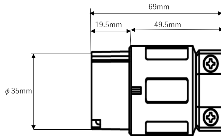
NEMA5-15R (メス)
