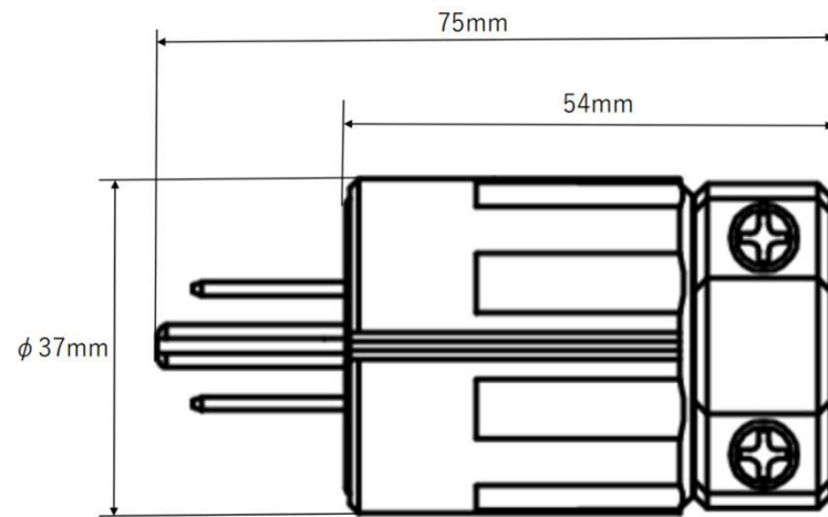
NEMA5-15P (オス)
